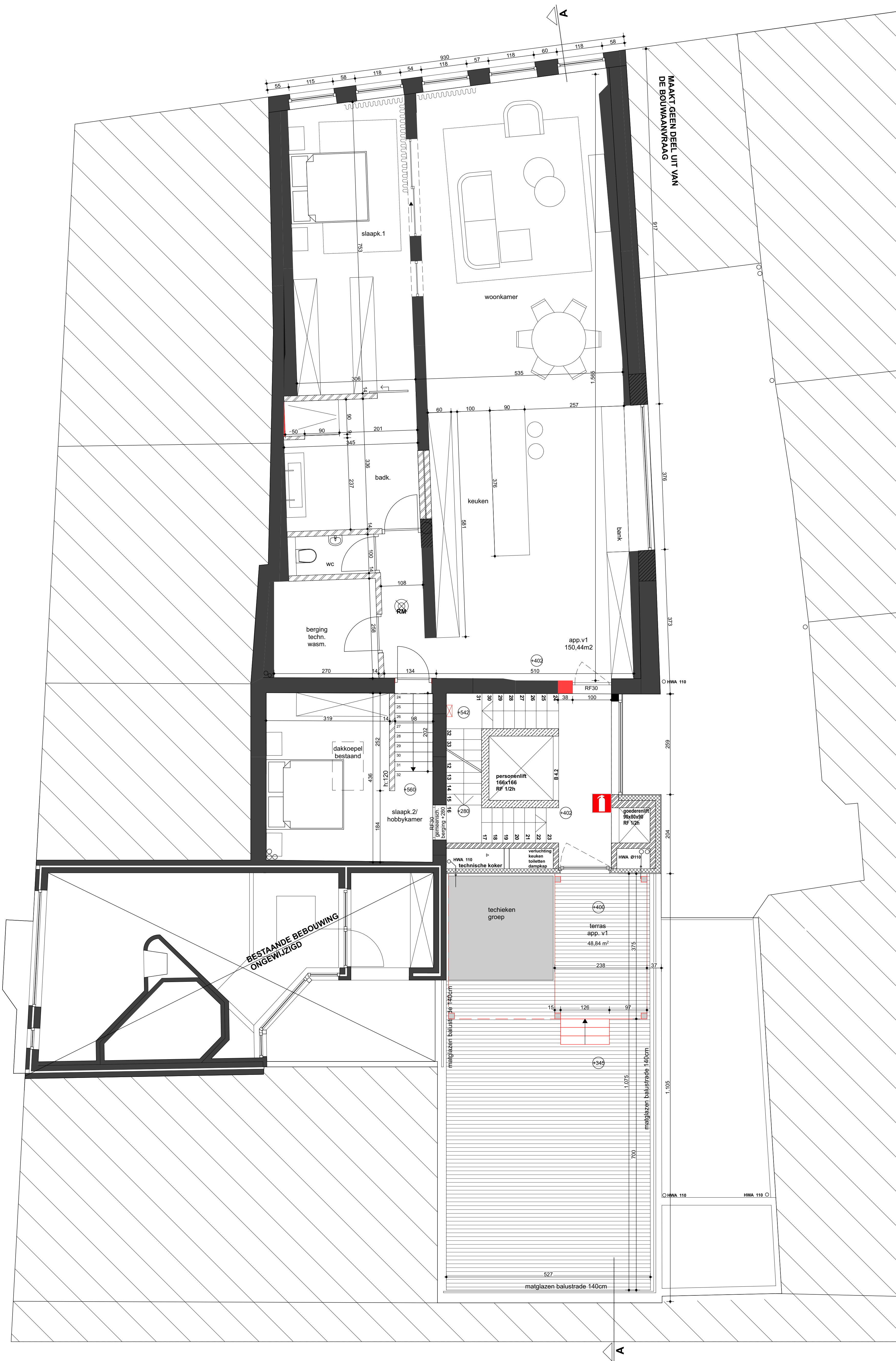
VERDIEPING 1
