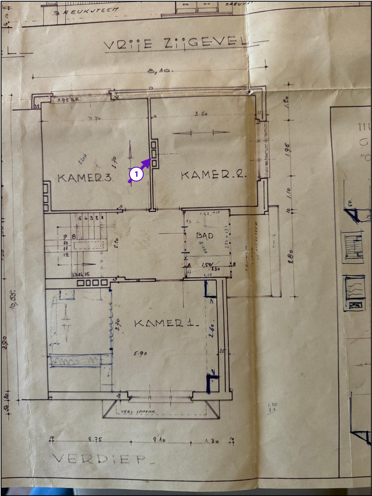
Legende van plan 1.5: Verdieping +1 kopie kopie
