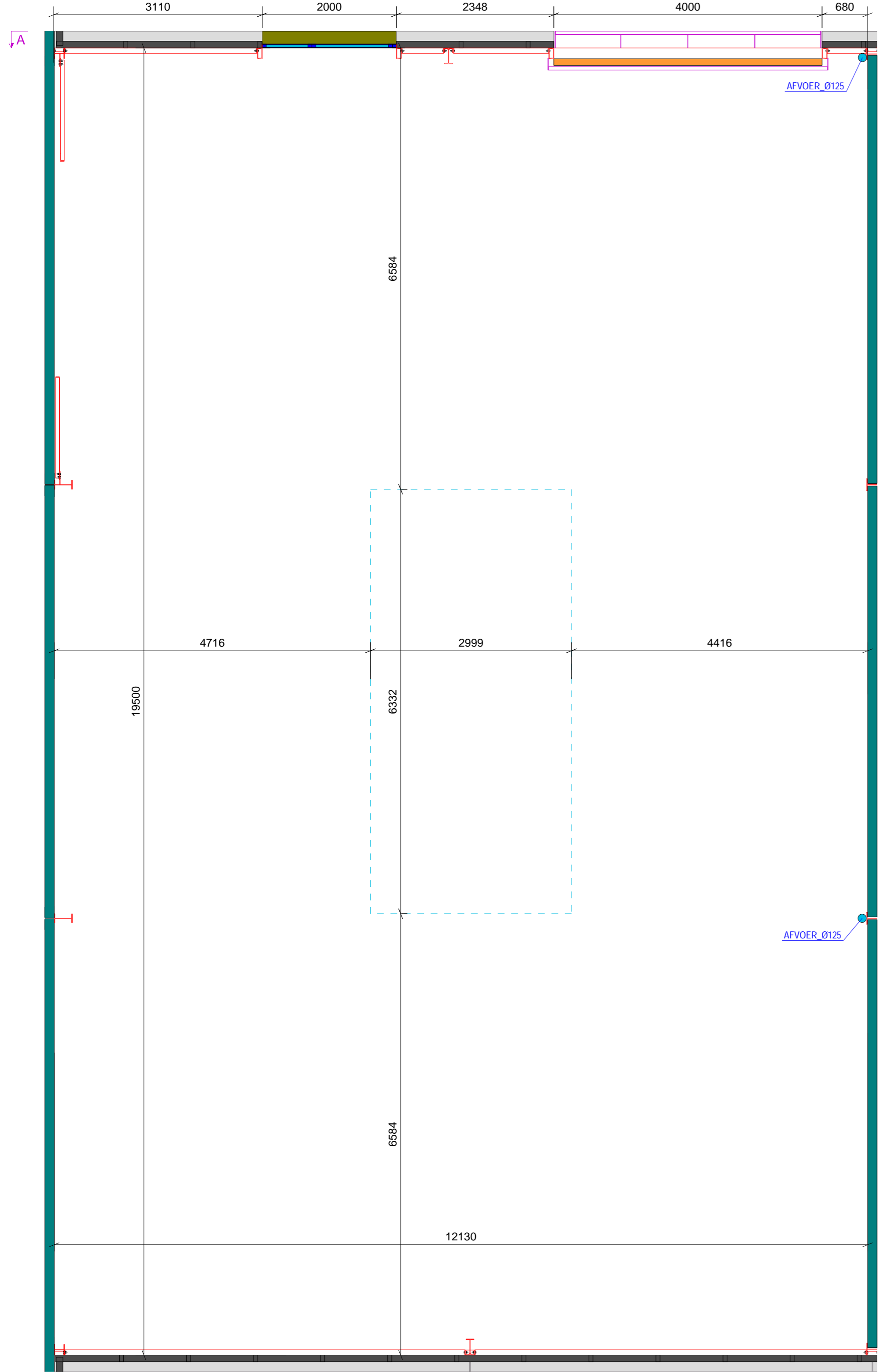
GELIJKVLOERS 1:50
